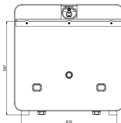
Oldalnézet
