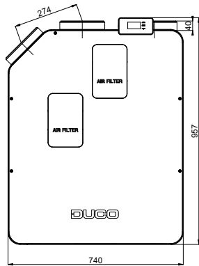
Előlnézet
