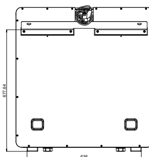
Hátnézet
