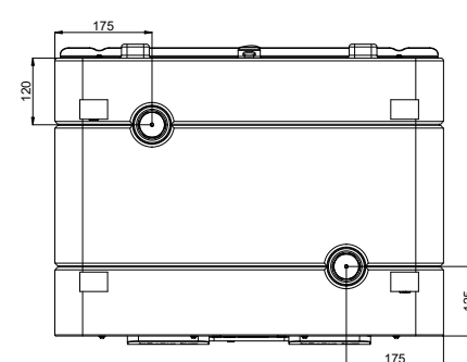
Alulnézet
