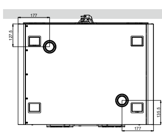
Alulnézet
