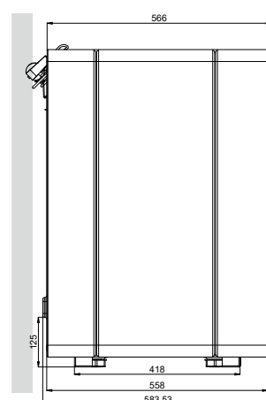
Oldalnézet
