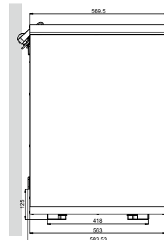
Oldalnézet
