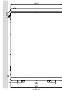
Oldalnézet
