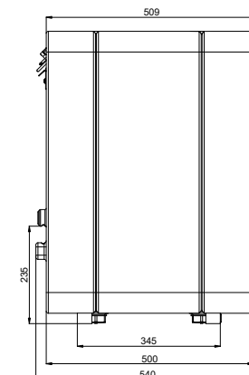
Oldalnézet
