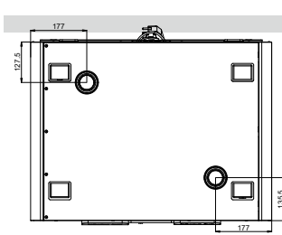
Alulnézet
