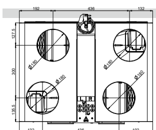
Oldalnézet
